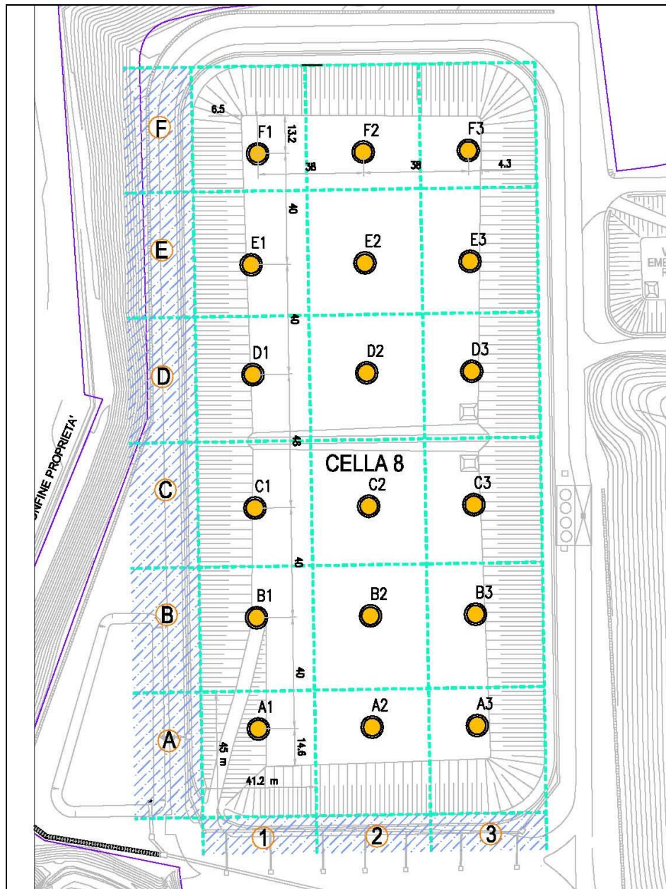
Figura 11 - Pozzetti di monitoraggio biogas nel corpo rifiuti
